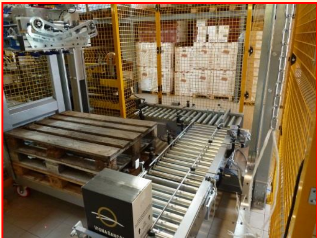
Trasportatori di deviazione ed accumulo scatole
